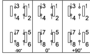
CSM02 Devre Şeması
