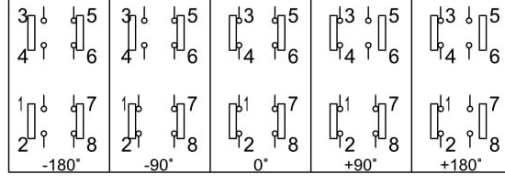
CSM04 Devre Şeması
