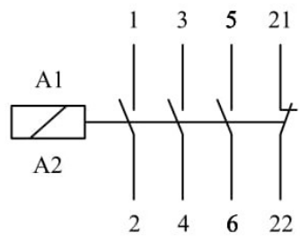
Elektrik Şeması
