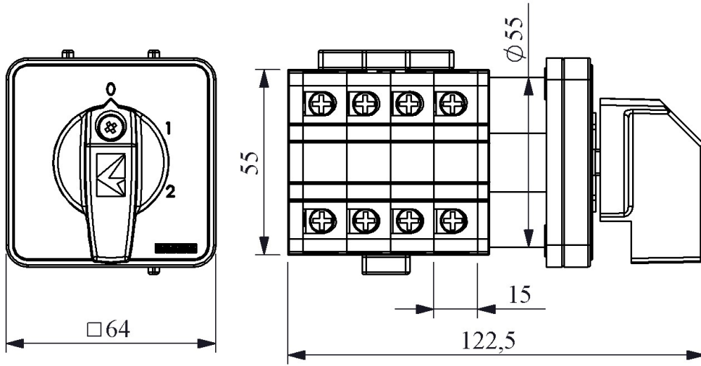
Devre Şeması
