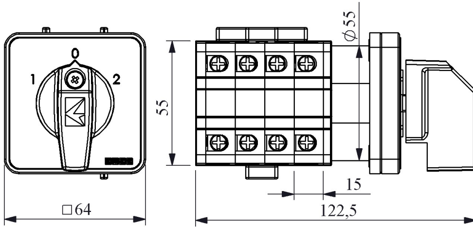
Devre Şeması
