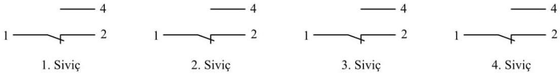
Devre Şeması
