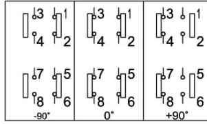
CSM02 Devre Şeması
