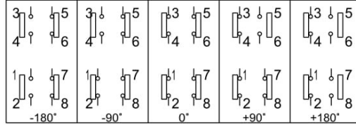
CSM04 Devre Şeması
