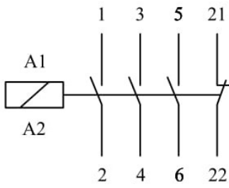
Elektrik Şeması
