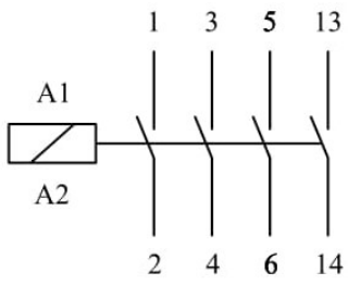
Elektrik Şeması
