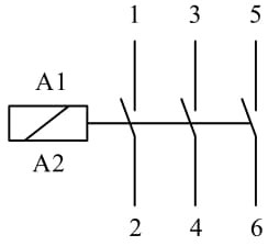
Elektrik Şeması
