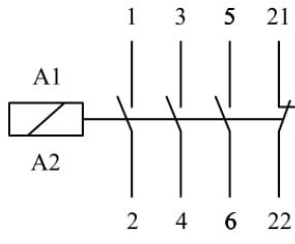
Elektrik Şeması
