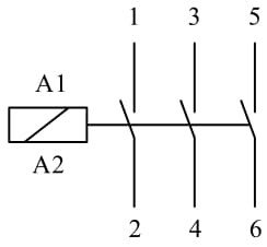
Elektrik Şeması
