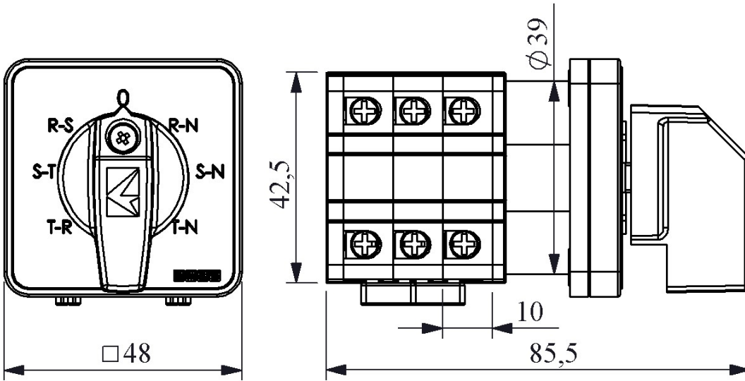
Devre Şeması
